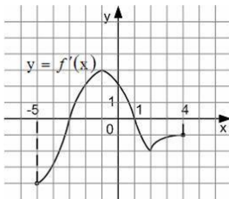
Рисунок. График производной функции y = f'(x)
